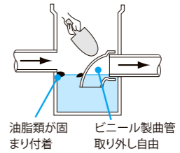
防臭ますの構造
