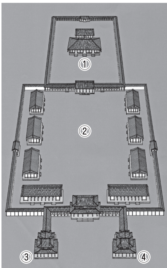
▲長岡宮朝堂院推定復原図
