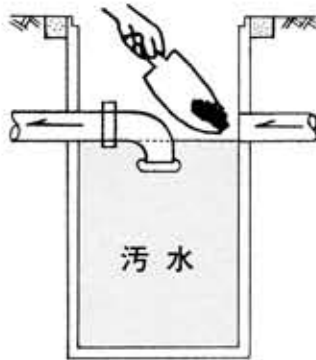
防臭ます構造図
