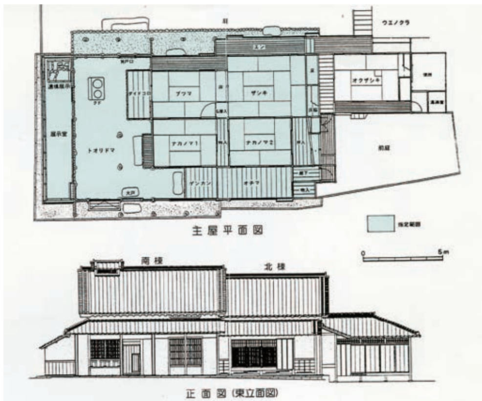
図 2-3-3-6 須田家住宅主屋平面図・正面図（東立面図）
