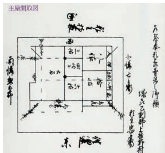
図 2-3-3-9 中小路家住宅 幕末の「主屋見取図」
