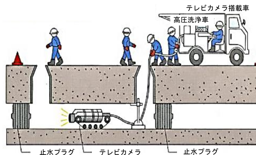
（図1）自走式テレビカメラ調査
