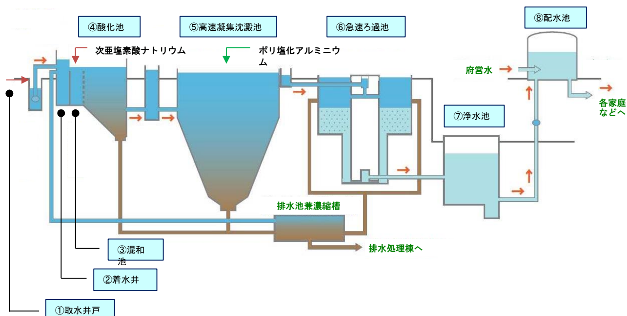
物集女西浄水場浄水処理工程フロー図
