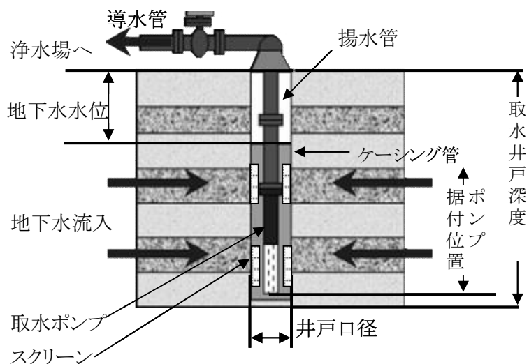
取水井戸の構造図
