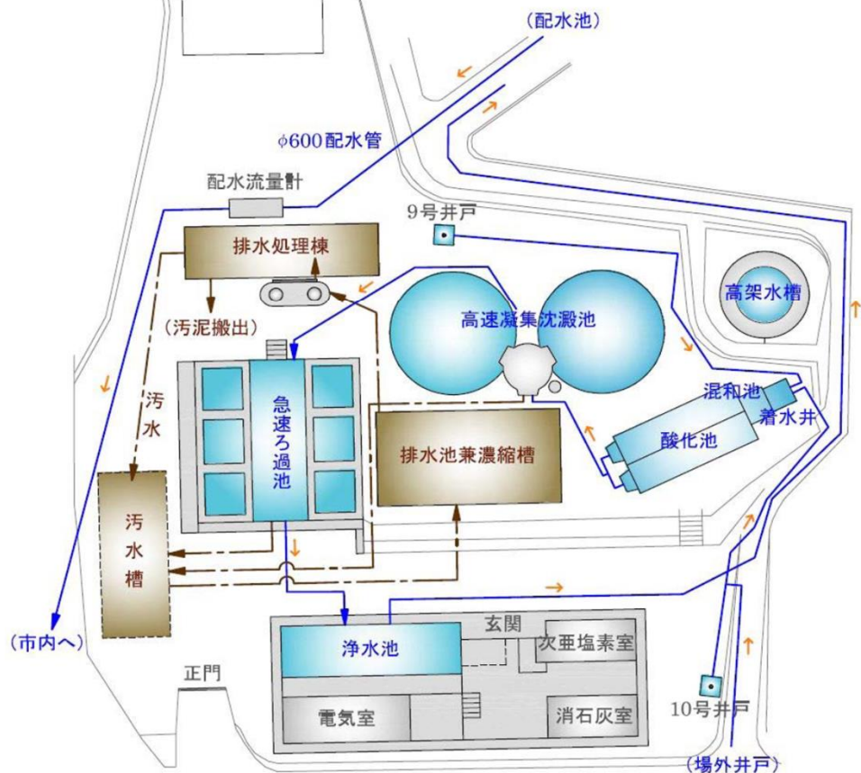
物集女西浄水場平面図
