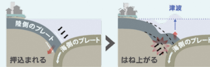
▲海溝(プレート境界)型地震のイメージ
