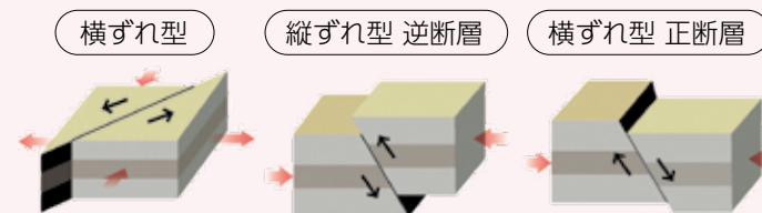
▲地盤のずれ方の違いによる断層の種類
