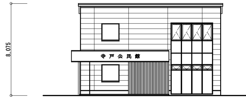
南側立面図
